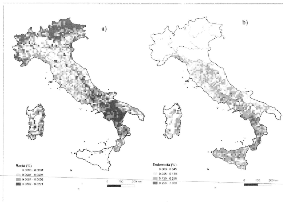
Figura 2 - Mappe della distribuzione sul territorio italiano della rarità (a) e dell'endemicità (b). I valori sono espressi in percentuale sul totale di specie in ogni cella. (Fonte: ISPRA "Rapporti Direttive Natura (2013-2018)")
