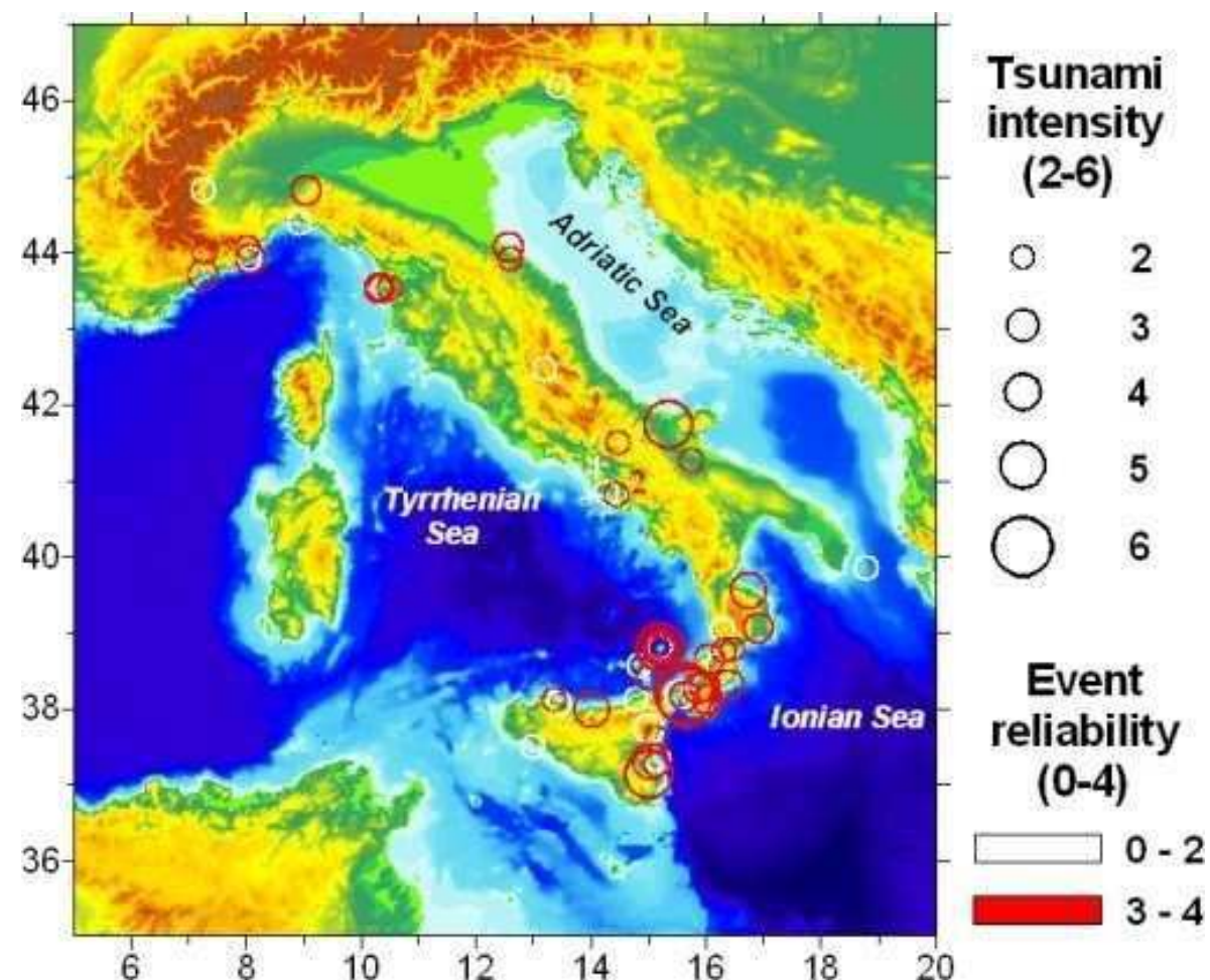
Figura 6.25 Maremoti avvenuti in Italia dal 79DC a oggi. Le dimensioni dei cerchi sono proporzionali all'intensità del maremoto, il colore all'affidabilità dell'evento.
