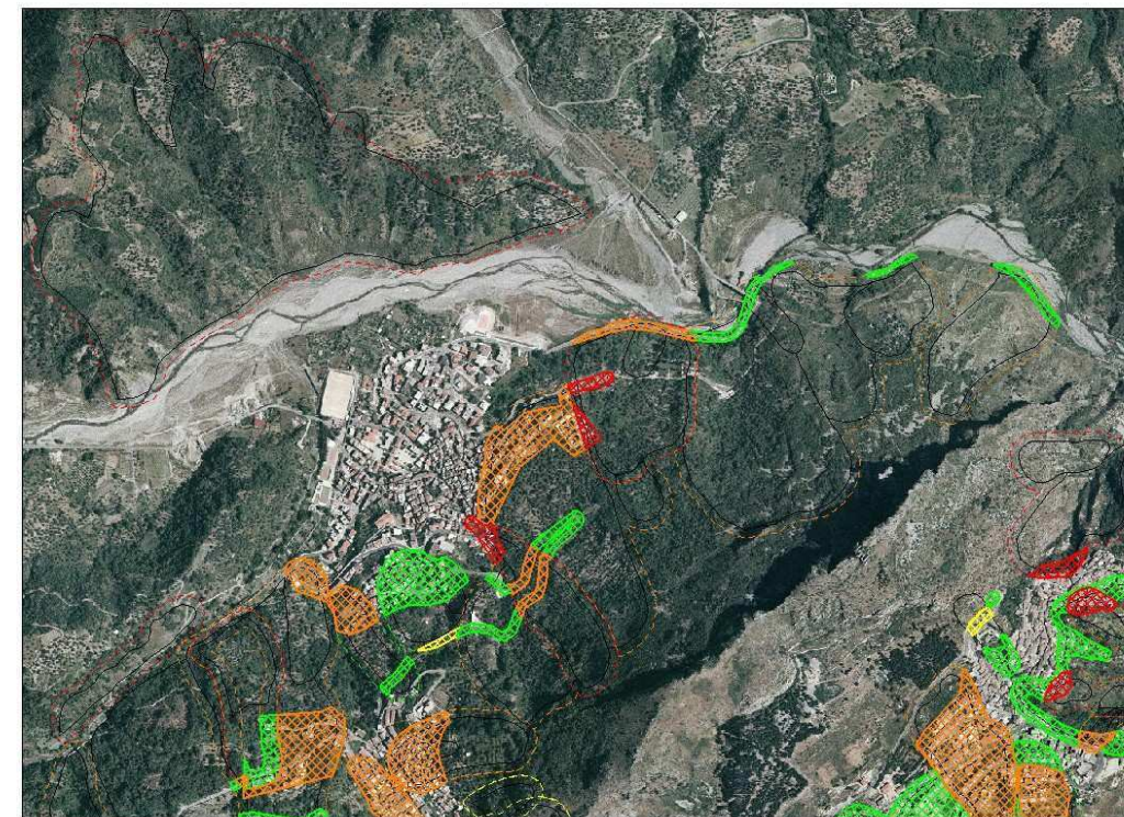
Figura 6.9 Areali di rischio Fonte: Autorità di Bacino della Regione Calabria.
