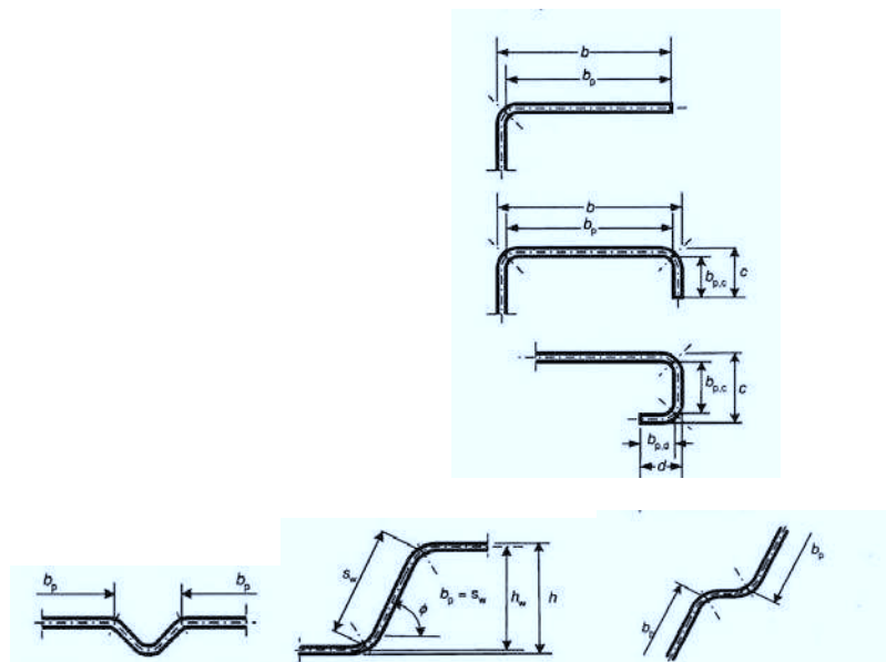
Figura C4.2.27 – Esempi di determinazione della larghezza b_p
